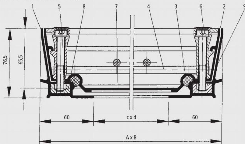
Type BVA Alu, Maštstab 1 : 2,5
